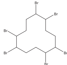
Hexabromocyclododecane (HBCD)
